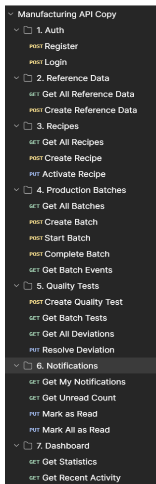
Рисунок 7 - Postman collection
