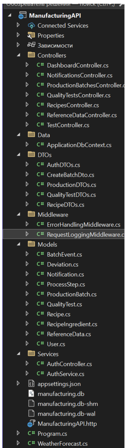
Рисунок 1 - Архитектура проекта
